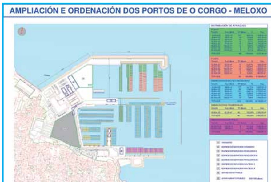
Planos da nova dársena do Corgo. Á esquerda, o director de Portos de Galicia.
